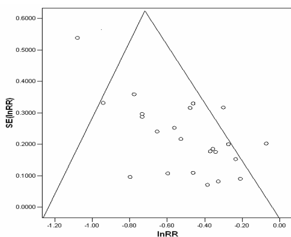
نمودار شماره ۱- نمودار فونل برای بررسی اربیی انتشار در برآورد لگاریتم میزان خطر نسبی مرگ در بیماران کرونری قلبی بعد از ترک سیگار
