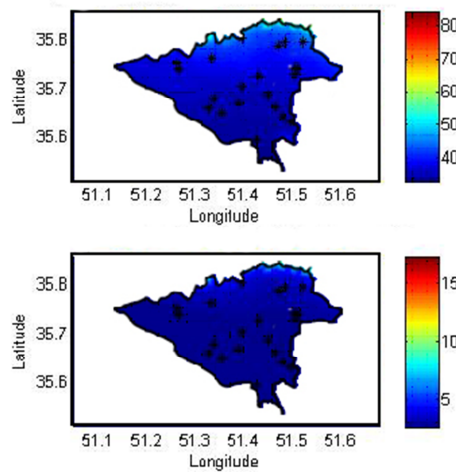
شکل شماره ۳- a: برآورد میانگین سالانه غلظت آلاینده دی‌اکسید نیتروژن در هوای شهر تهران در سال ۲۰۱۴ و b: برآورد خطای معیار آلاینده دی‌اکسید نیتروژن در هوای شهر تهران در سال ۲۰۱۴. (ایستگاه‌های سنجش آلاینده با علامت ستاره نشان داده شده است).
