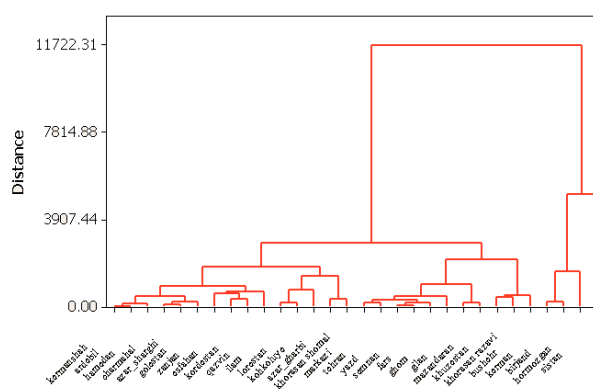
نمودار شماره ۱- نمودار دندوگرام از ساختار خوشه‌بندی استان‌ها
